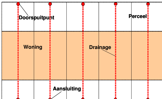
Figuur 3: Ligging drainage bij geschakelde/aaneengesloten bebouwing
