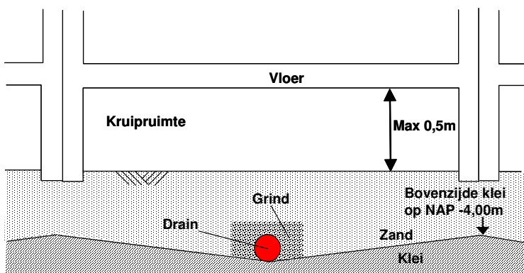
Figuur 4: Dwarsdoorsnede drainage bij geschakelde/aaneengesloten bebouwing
