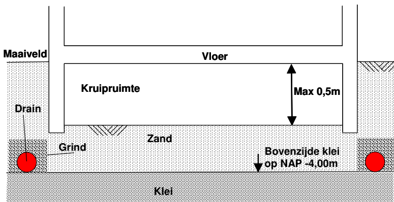
Figuur 2: Dwarsdoorsnede drainage bij vrijstaande/twee-onder-een-kap bebouwing
