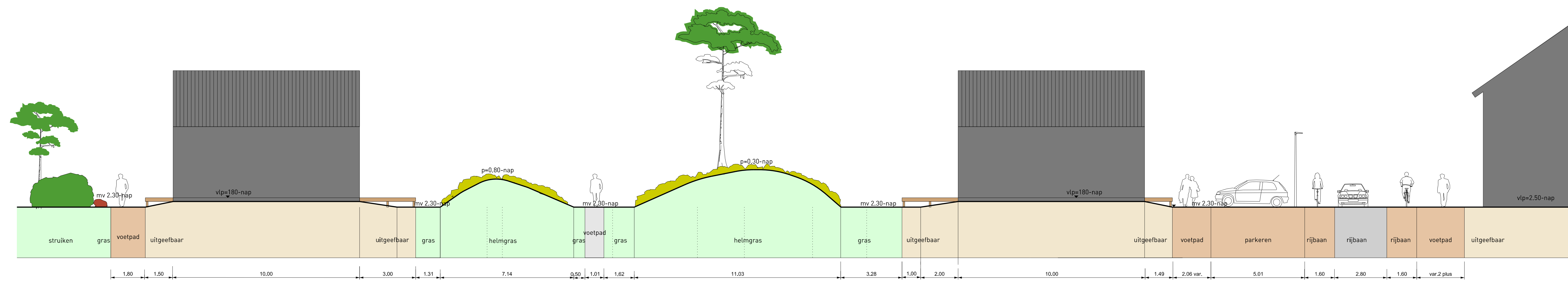
PROFIEL KLEINER WONEN schaal 1:100
